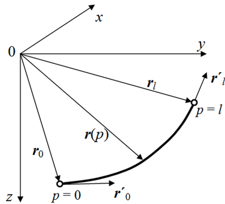
Рис. 2. Осевая линия элемента ГС
