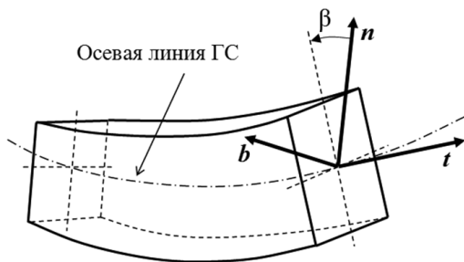
Рис. 3. Поворот конечного поперечного сечения элемента ГС относительно нормали репера Френе осевой линии, состоящего из вектора касательной t , нормали n и бинормали b
